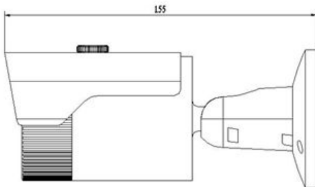
ZPI132/ZPI132P
